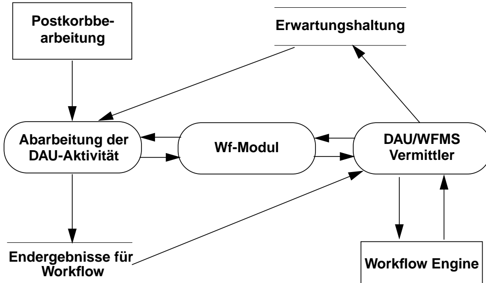
Abbildung 7: reaktiver Planer/WFMS
