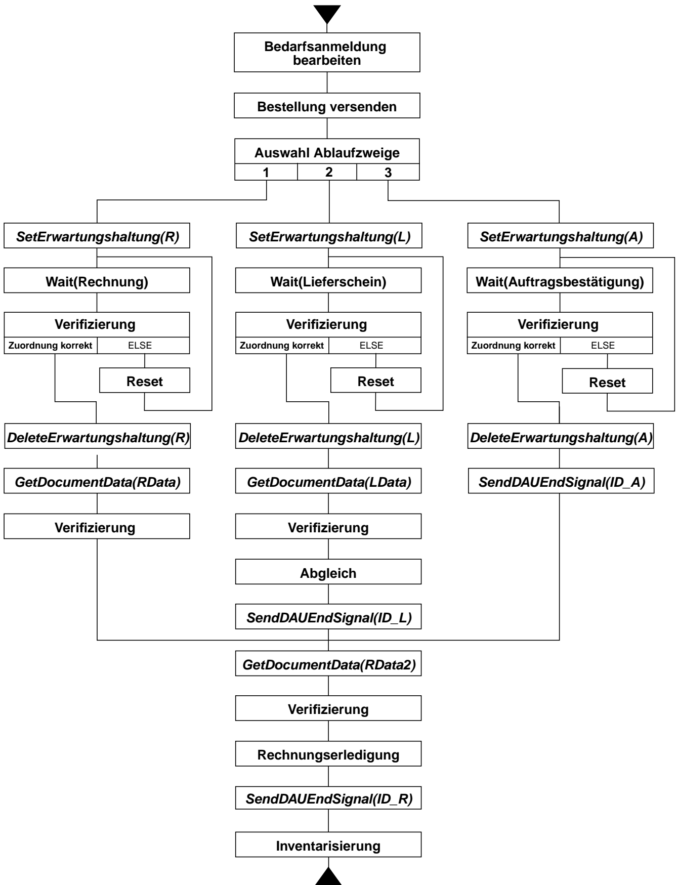
Abbildung 5: Workflow-Definition Bestellung
