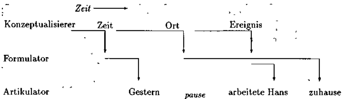
Abbildung 2: Inkrementelle Generierung.
