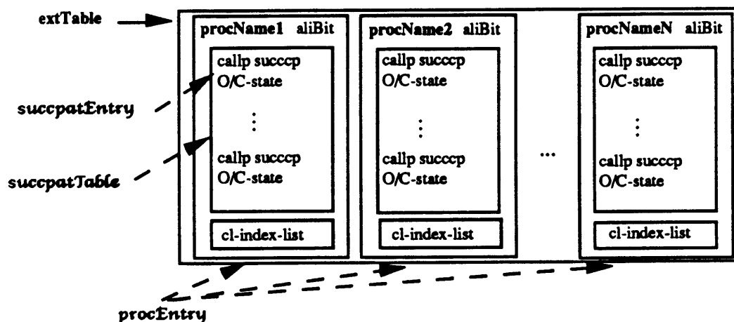
Bild 3.5 Zentrale Datenstruktur extension table ( extTable ) des mode-Interpreters
