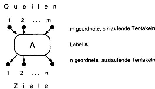
Abbildung 2.6: Hyperkante
