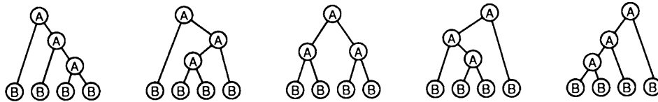
Abbildung 3.8: Die fünf möglichen Binärbäume (Parse) für n = 4 , ohne Permutationen
